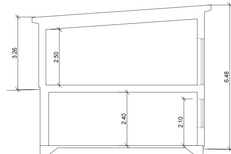
SEKTION A-A
