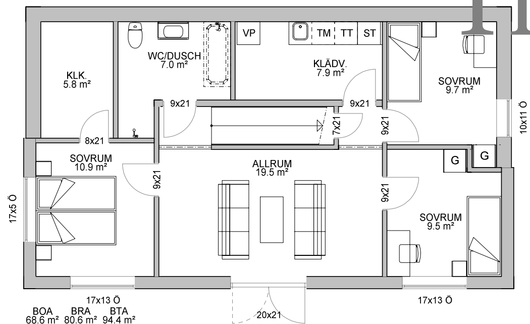
SLUTTNINGSPLAN
