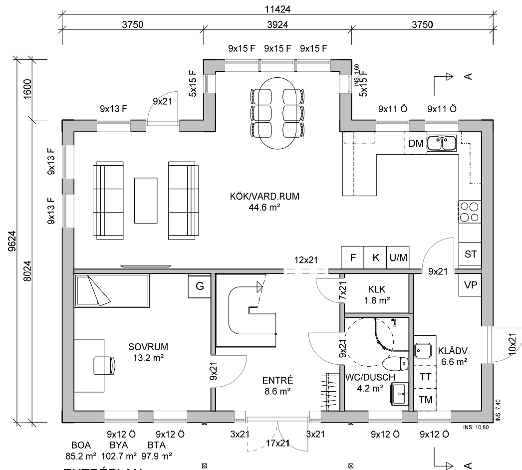
ENTRÉPLAN
