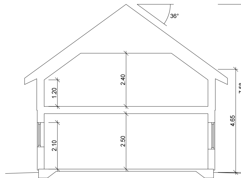
SEKTION A-A
