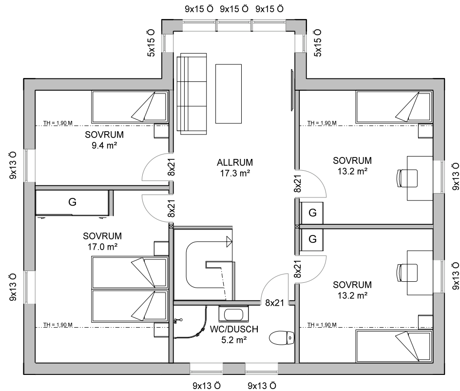
ÖVRE PLAN
